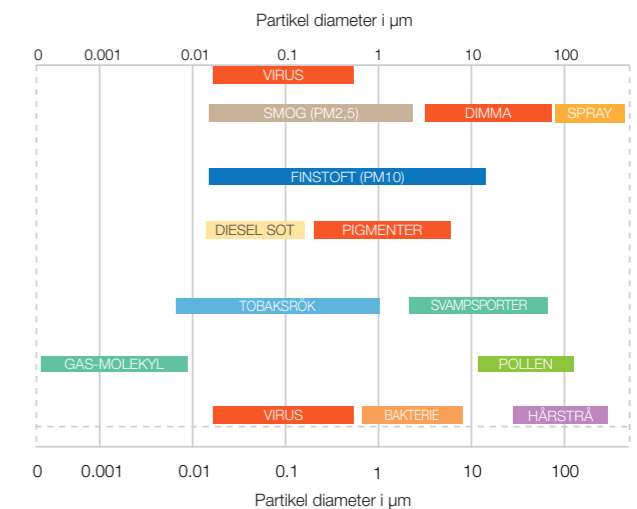
Grafik1: Storleksjämförelse av fasta och gasformiga ämnen i den omgivande luften.
